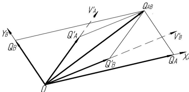
Рис. 3.4. Диаграмма векторов количества движения
