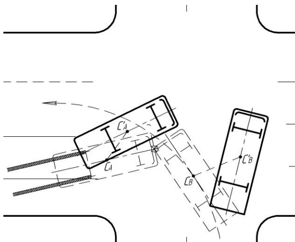
Рис. 3.2. Пример схемы столкновения на перекрёстке: Сплошные линии – ТС после столкновения, штриховые – в момент первого контакта
