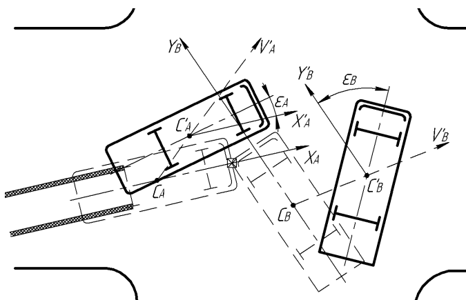
Рис. 3.3. Схема столкновения автомобилей для расчета по графическому методу
