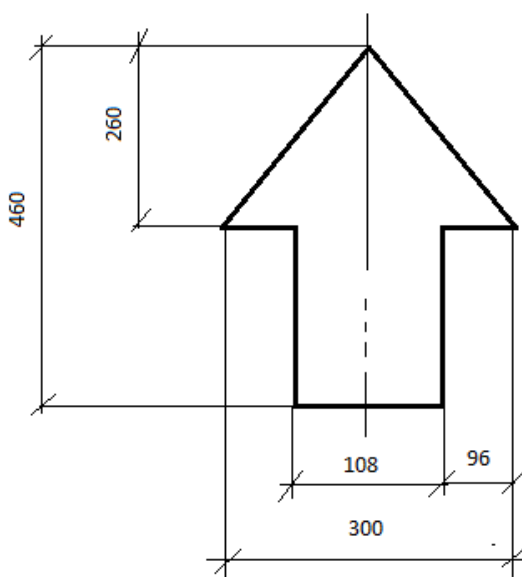
Рисунок 1.1.1 Размеры стрелки
