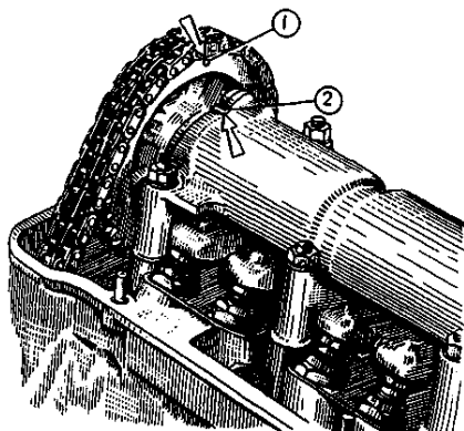
Рис. 2.15. Проверка совпадения установочной метки на звездочке распределительного вала с меткой на корпусе подшипников: 1 – метка па звездочке; 2 – метка на корпусе подшипников
