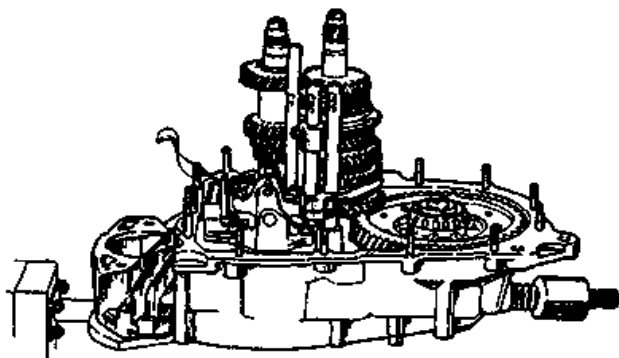
Рис. 3.12. Установка штоков и вилок переключения передач
