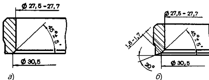
Рис. 2.24. Профиль седла выпускного клапана: а – новое седло; б – седло после ремонта
