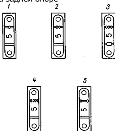
Рис. 2.11. Установка упорных полуколец на задней опоре
