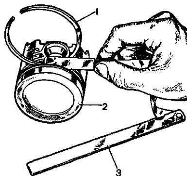
Рис. 2.40. Проверка зазора между поршневыми кольцами и канавками: 1 – поршневое кольцо; 2 – поршень; 3 – набор щупов
