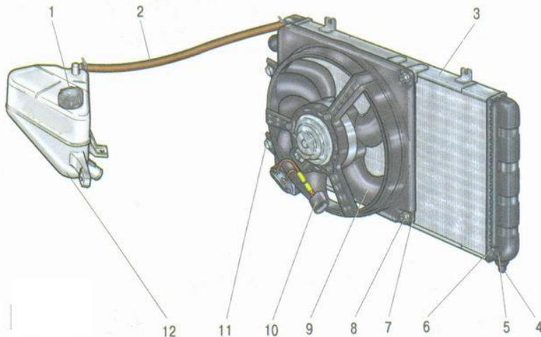
Рис. 1.24. Радиатор с электровентилятором и расширительный бачок: 1 – пробка расширительного бачка; 2 – пароотводящий шланг; 3 – радиатор; 4 – подушка опоры радиатора; 5 –
