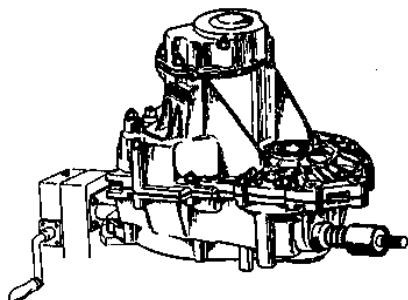
Рис. 3.1. Коробка передач, установленная на стенде для разборочно-сборочных работ
