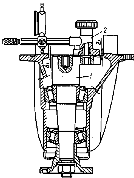
Рис. 4.15. Схема снятия замеров для определения толщины регулировочного кольца ведущей шестерни: 1 – оправка А.70184; 2 – приспособление А.95690 с индикатором; a_1 и a_2 – расстояния
