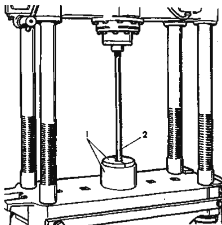
Рис. 4.7. Выпрессовка запорного кольца подшипника полуоси приспособлением А.74108/R:
