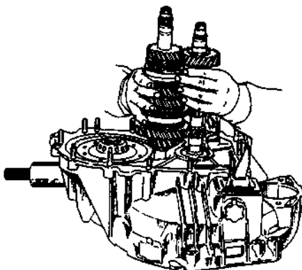
Рис. 3.5. Снятие первичного
