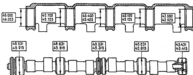
Рис. 2.29. Основные размеры распределительного вала и корпуса подшипников
