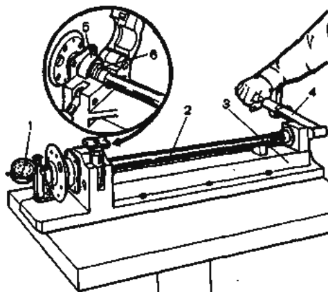
Рис. 4.9. Проверка усилия, с которым выпрессовывается запорное кольцо подшипника полуоси, с помощью приспособления А.95601/R и динамометрического ключа: 1 – индикатор; 2 – полуось; 3 – приспособление А.95601/R; 4 – динамометрический ключ; 5 – шарикоподшипник; 6 – запорное кольцо подшипника
