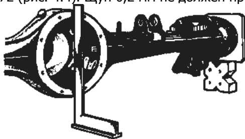
Рис. 4.4. Проверка перпендикулярности поверхности крепления редуктора
