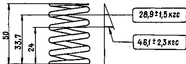
Рис. 2.25. Основные данные для проверки наружной пружины клапана
