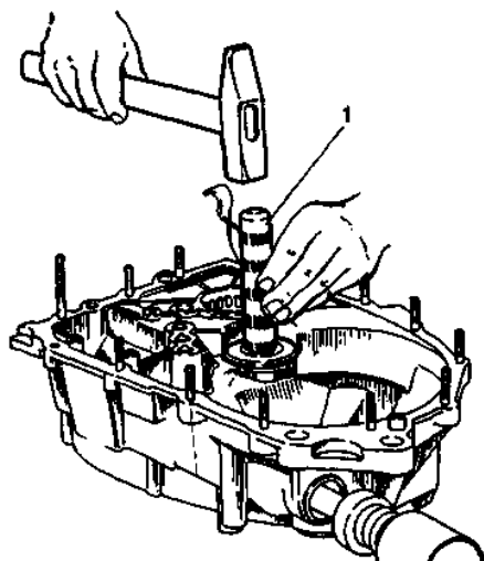
Рис. 3.11. Запрессовка подшипника вторичного вала: 1 – оправка 67.7853.9574
