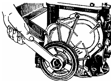
Рис. 2.2. Отворачивание гайки коленчатого вала ключом А.50121
