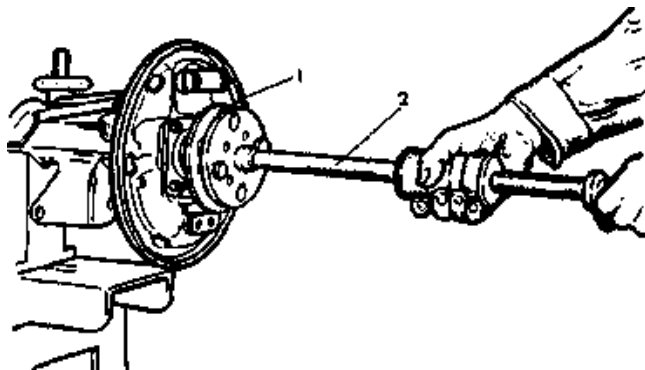
Рис. 4.1. Выпрессовка полуоси с помощью съёмника 67.7801.9516:
