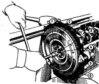
Рис. 2.7. Снятие маховика: 1 – ключ; 2 – маховик; 3 – болт крепления маховика; 4 – шайба; 5 – фиксатор А.60330/R для удержания маховика от проворачивания; 6 – передняя крышка картера сцепления
