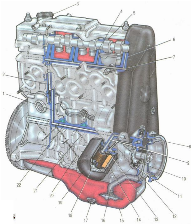
Рис. 1.22. Система смазки двигателя
