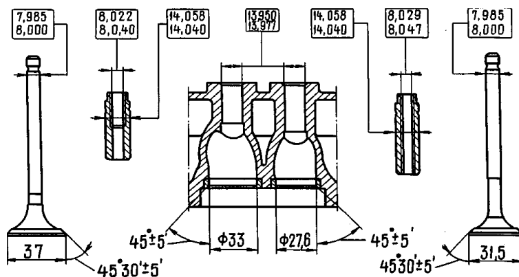
Рис. 2.20. Основные размеры клапанов, направляющих втулок и седел клапанов
