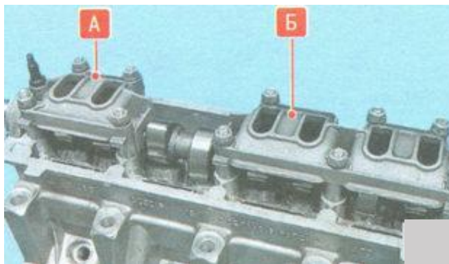
Рис. 1.25. Гайки крепления переднего А и заднего Б корпусов подшипников распределительного вала
