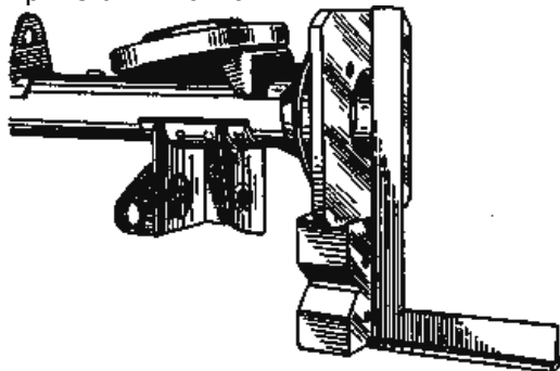
Рис. 4.2. Проверка деформаций балки заднего моста с помощью угольника по наружной поверхности фланца А.70172
