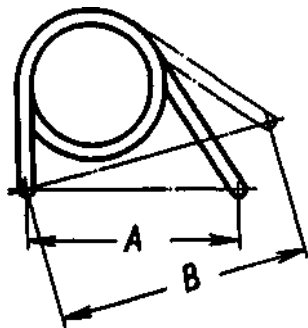
Рис. 2.27. Схема проверки пружины рычага: А – размер в свободном состоянии; В – размер под нагрузкой
