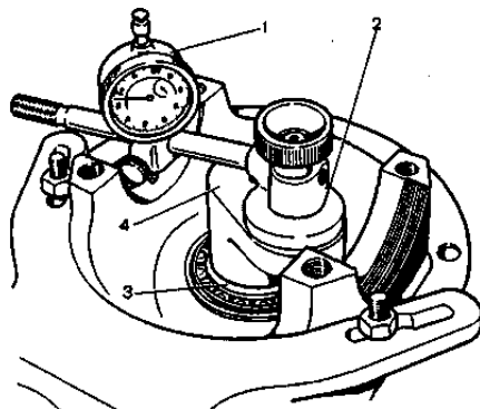
Рис. 4.14. Определение толщины регулировочного кольца
