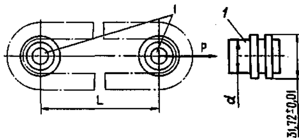
Рис. 2.34. Схема проверки износа (вытяжки) цепи: 1 – ролики
