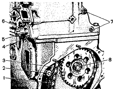
Рис. 2.3. Снятие натяжителя и успокоителя цепи:
