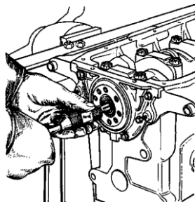
Рис. 2.8. Выпрессовывание подшипника вала коробки передач из коленчатого вала выталкивателем А.40006
