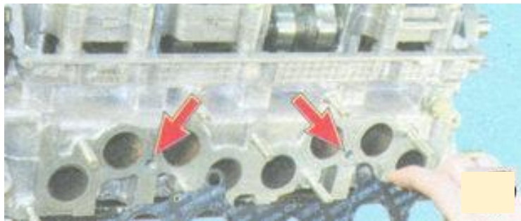
Рис. 1.29. Технологические каналы водяной рубашки головки блока цилиндров
