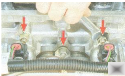
Рис. 1.6. Три верхние гайки крепления впускного коллектора и катколлектора
