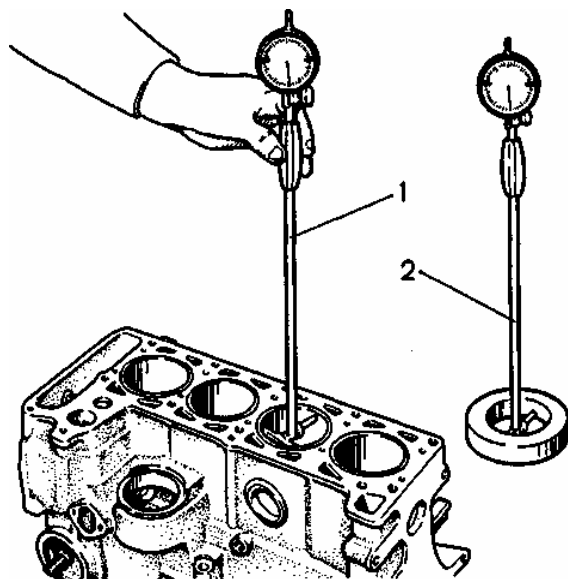
Рис. 2.18. Измерение цилиндров нутромером: 1 – нутромер; 2 – установка нутромера на ноль по калибру 67.8125.9501
