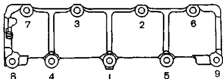
Рис. 2.16. Порядок затягивания гаек корпуса подшипников распределительного вала
