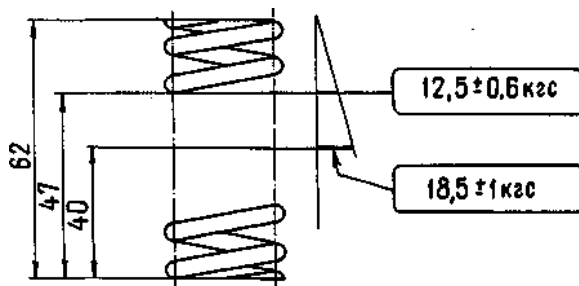
Рис. 2.32. Основные данные для проверки пружины натяжителя
