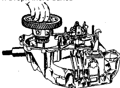
Рис. 3.6. Снятие дифференциала
