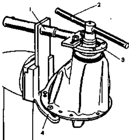
Рис. 4.11. Отвертывание самоконтрящейся гайки ведущей шестерни: 1 – стопор для фиксирования фланца ведущей шестерни; 2 – торцовый ключ; 3 – фланец ведущей шестерни; 4 – кронштейн для крепления редуктора на стенде
