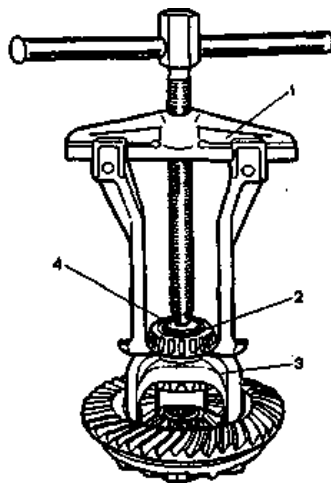
Рис. 4.13. Снятие внутреннего кольца подшипника коробки дифференциала универсальным съемником А.40005/1/6: 1 – универсальный съемник А.40005/1/6; 2 – внутреннее кольцо подшипника; 3 – коробка дифференциала; 4 – упор А.45028
