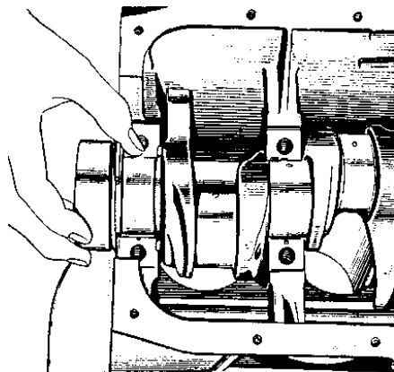
Рис. 2.11. Установка упорных полуколец на задней опоре
