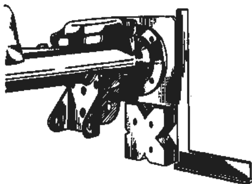
Рис. 4.3. Проверка скручивания балки заднего моста с помощью угольника по боковой поверхности фланца А.70172
