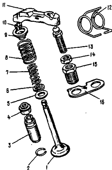
Рис. 2.9. Детали клапанного механизма: 1 – клапан; 2 – стопорное кольцо; 3 – направляющая втулка; 4 – маслоотражательный колпачок; 5 – опорная шайба наружной пружины; 6 – стопорная шайба внутренней пружины; 7 – внутренняя пружина; 8 – наружная пружина; 9 – тарелка пружин; 10 – сухари; 11 – рычаг привода клапана; 12 – пружина рычага; 13 – регулировочный болт; 14 – контргайка регулировочного болта; 15 – втулка регулировочного болта; 16 – стопорная пластина пружины рычага
