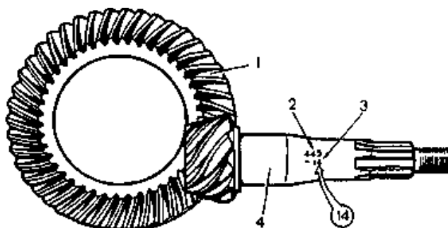
Рис. 4.16. Шестерни главной передачи: 1 – ведомая шестерня; 2 – порядковый номер; 3 – поправка в сотых долях миллиметра к номинальному положению; 4 – ведущая шестерня
