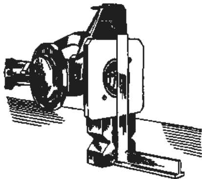
Рис. 4.5. Проверка горизонтальных деформаций балки заднего моста с помощью угольника по наружной поверхности фланца А70172
