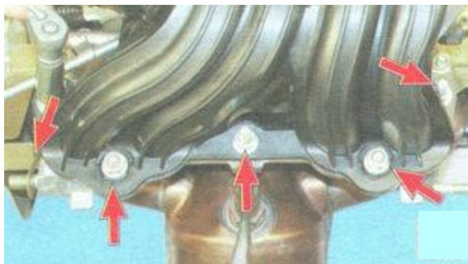
Рис. 1.1. Гайки крепления модуля впуска к впускному коллектору
