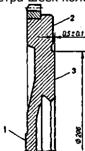
Рис. 2.37. Маховик:
