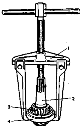
Рис. 4.12. Снятие внутреннего кольца заднего подшипника ведущей шестерни универсальным съемником А.40005/1/7: 1 – универсальный съемник А.40005/1/7; 2 – ведущая шестерня; 3 – внутреннее кольцо подшипника; 4 – приспособление А.45008
