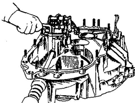
Рис. 3.7. Снятие механизма выбора передач
