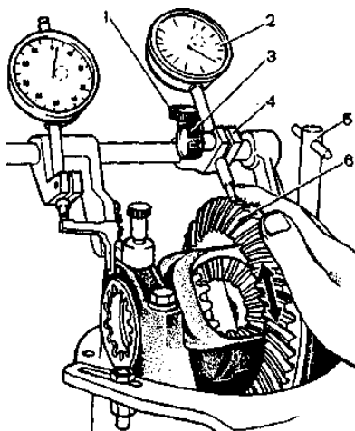
Рис. 4.19. Проверка бокового зазора в зацеплении шестерен главной передачи приспособлением А.95688/Р: 1 – винт затягивания кронштейна; 2 – индикатор для проверки бокового зазора в зацеплении ведущей и ведомой шестерен; 3 – винт крепления стержня индикатора; 4 – кронштейн индикатора; 5 – винт крепления; 6 – ведомая шестерня
