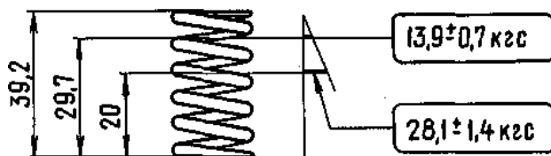
Рис. 2.26. Основные данные для проверки внутренней пружины клапана
