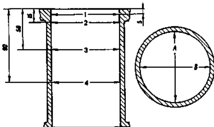
Рис. 2.19. Схема измерения цилиндров: А и В – направления измерений; 1 – 4 – номера поясов
