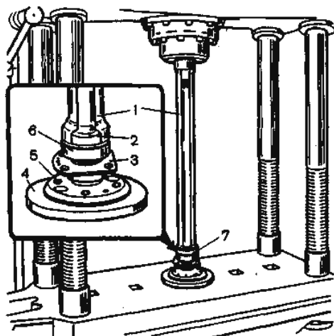
Рис. 4.8. Запрессовка запорного кольца подшипника полуоси: 1 – оправка А.74107/ 2R; 2 – запорное кольцо подшипника; 3 – пластина крепления подшипника и маслоотражатель в сборе с прокладкой; 4 – опорное кольцо А.74107/1R; 5 – полуось; 6 – подшипник; 7 – обойма А.74107/4R
