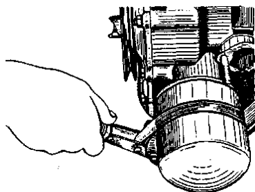
Рис. 2.1. Снятие масляного фильтра приспособлением А. 60312
