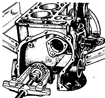
Рис. 2.6. Снятие звездочки коленчатого вала универсальным съемником
