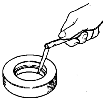
Рис. 2.41. Проверка зазора в замке колец
