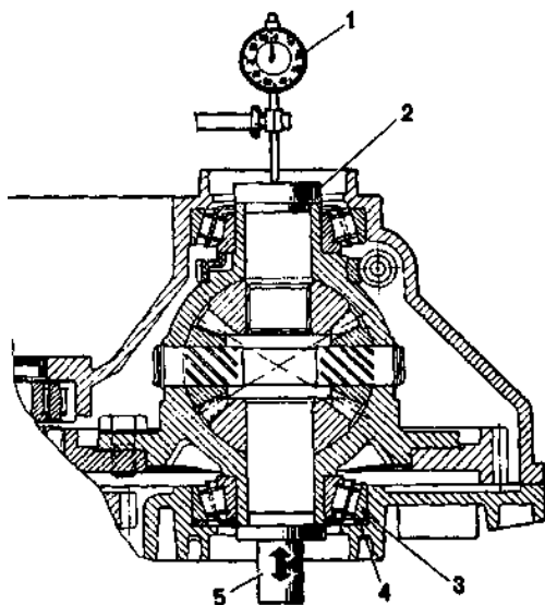
Рис. 3.13. Схема подбора толщины регулировочного кольца подшипников дифференциала: 1 – индикатор; 2 – опорная оправка; 3 – подшипник дифференциала; 4 – установочное кольцо (имеет постоянную толщину, равную 1,25 мм); 5 – оправка
