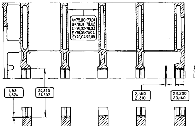
Рис. 2.17. Основные размеры блока цилиндров
