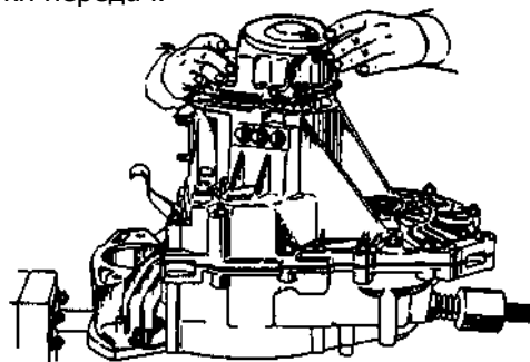
Рис. 3.2. Снятие задней крышки картера коробки передач
