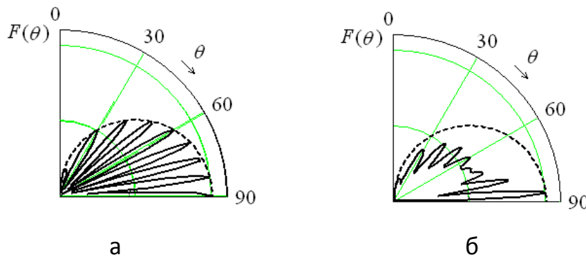
Рисунок 15.3 – Влияние свойств отражающей поверхности на диаграмму направленности электрического вибратора
