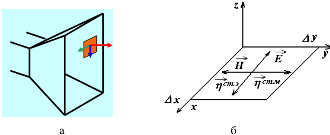
Рисунок 5.3 – Введение элемента Гюйгенса
