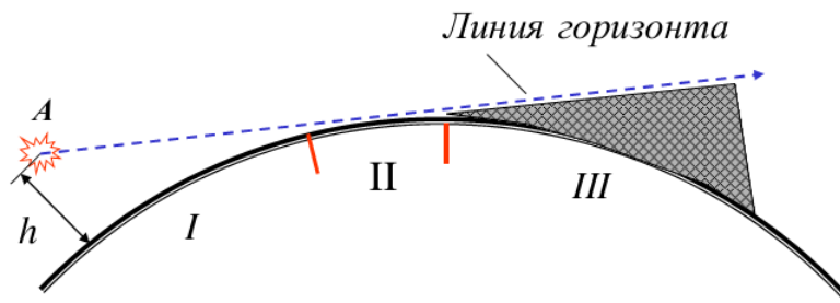
Рисунок 14.2 – Пояснение областей освещенности
