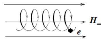
Рисунок 17.1 – Движение электронов вокруг силовых линий Земли
