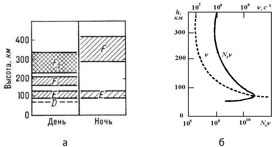
Рисунок 17.2 – Структура ионосферы
