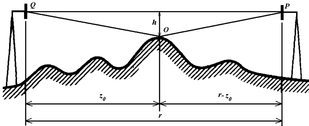
Рисунок 14.7 – Геометрия задачи определения типа трассы
