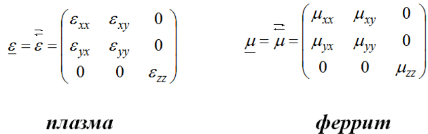
Рисунок 6.2 – Частный случай анизотропных сред – гиротропные среды
