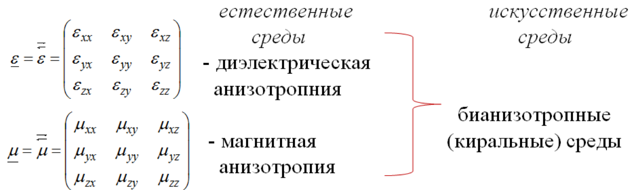
Рисунок 6.1 – Разделение анизотропных сред
