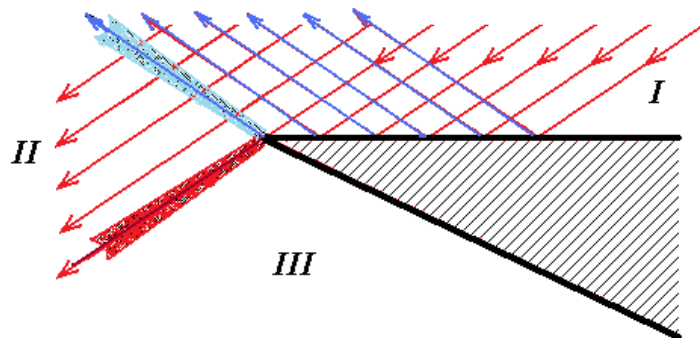
Рисунок 12.4 – Создаваемые области в задаче дифракции волны на клине
