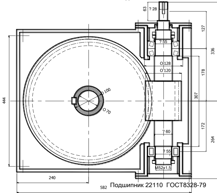
Рисунок 21. Компонка редуктора с вертикальной осью вращения на выходе и полым тихоходным валом
