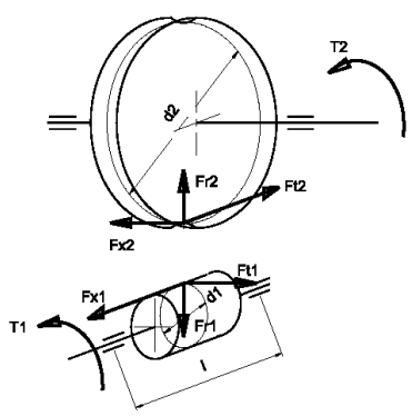
Рис. 8. Силы в зацеплении червячной передачи
