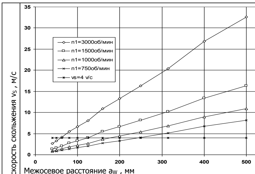
Рис. 6. Осредненные скорости скольжения v_s , м/с, для передаточных чисел 8..80, в диапазоне межосевых расстояний a_w 40..500 мм при частотах вращения червяка n_1 750..1500 об/мин. Наибольшее отклонение v_s при максимальных передаточных числах до 8 %.
