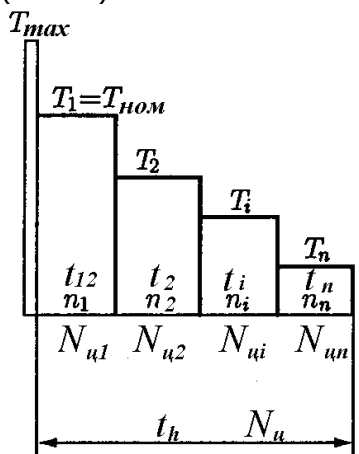
Рис. 3. Циклограммы нагрузки на валах привода
