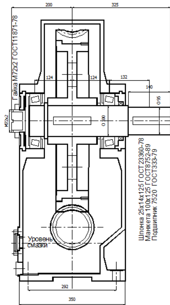
Рисунок П.1. Компонка редуктора с горизонтальными валами и нижним расположением червяка
