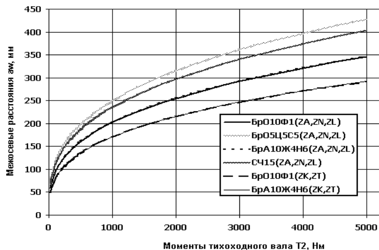
Рис. П.2. Межосевые расстояний червячных передач по условию контактной выносливости для червячных колес из материалов 1, 2 и 3 групп в сочетании с линейчатыми (ZA, ZN, ZL, ZK) и нелинейчатыми (ZT) червяками при непрерывном режиме работы
