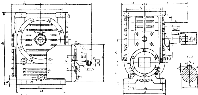
Рис.16. Редуктор червячный одноступенчатый типа Ч ( a_w 50, 60, 80, 100, 125, 160) ГОСТ27701-88. Вал тихоходный в сборе с ко-
