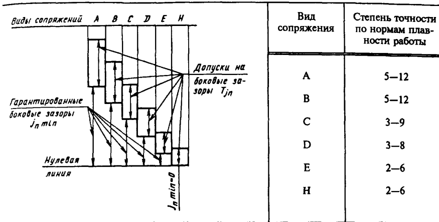
Рис. 7. Виды сопряжений поверхностей зубьев червячных колес и витков червяка.
