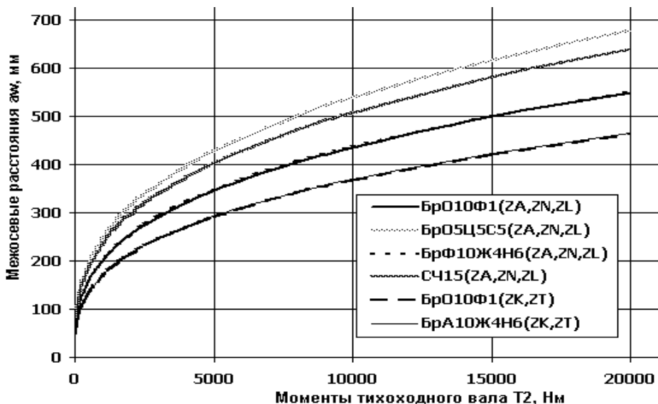
Рис. 8. Межосевые расстояния червячных передач по условию контактной выносливости для червячных колес из материалов 1, 2 и 3 групп в сочетании с линейчатыми (2А, 2N, 2L) и нелинейчатыми (2К, 2Т) червяками при непрерывном режиме работы.
