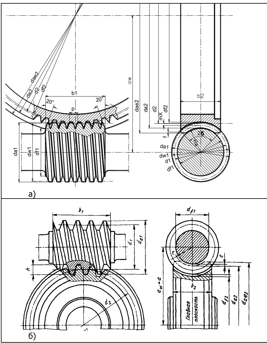
Рис. 5. Геометрические параметры червячных передач а) с коэффициентом смещения X = 0,714 ; б) с коэффициентом смещения X = 0 [1, Т.2, гл.4] .
