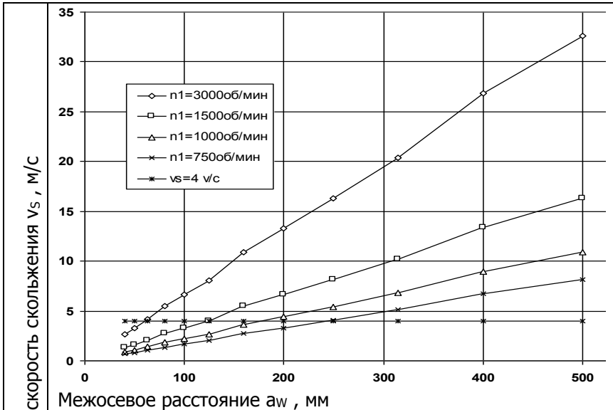
Рис. 6 (дубль). Осредненные скорости скольжения v_s , м/с, для передаточных чисел 8..80, в диапазоне межосевых расстояний a_w 40..500 мм при частотах вращения червяка n_1 750..1500 об/мин. Наибольшее отклонение v_s при максимальных передаточных числах до 8 %.
