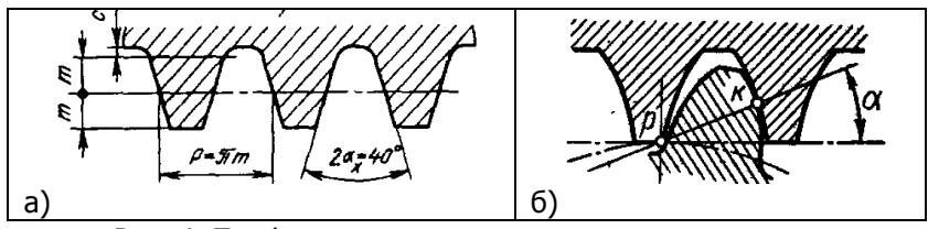
Рис. 4. Профили витков червяков в осевом сечении
