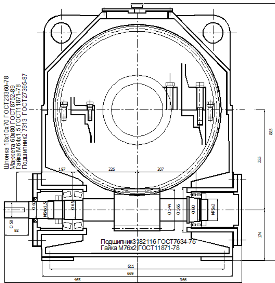
Рисунок П.1. Компонка редуктора с горизонтальными валами и нижним расположением червяка
