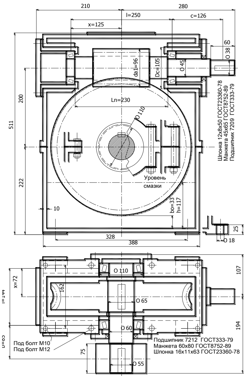
Рисунок 20. Компоновка редуктора с горизонтальными валами и верхним расположением червяка
