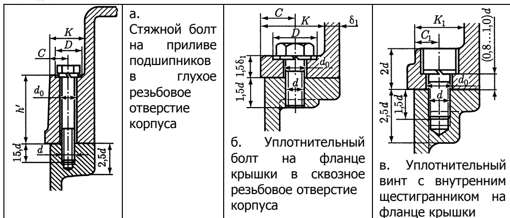
Рис. 18. Резьбовые соединения корпуса и крышки редуктора по плоскости разъема. Размеры конструктивных элементов:
