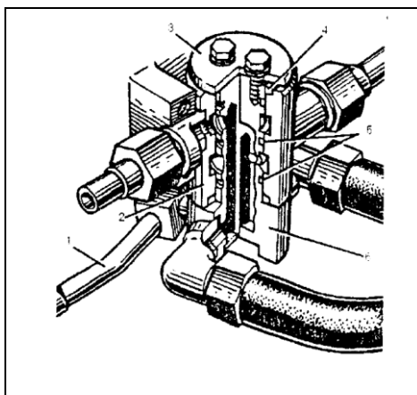
Рис.2 Гидропереход: 1 – поводок; 2 – корпус; 4,5 – уплотнительные кольца; 6 – ось
