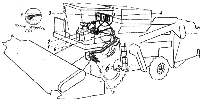
Рис.2 - Схема расположения ходовой гидросистемы комбайна «Дон 1500Б»: 1 - аксиально-плунжерный насос НП-90; 2 - масляный радиатор; 3 - бак; 4 - фильтр; 5 - аксиально-плунжерный мотор МП-90; 6 -заправочная муфта.
