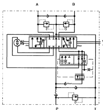
Рис.3 Насос-дозатор моноблочный
