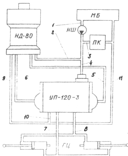
Рис.2 - Схема гидросистемы рулевого управления: 1 – магистраль всасывания, 2, 3 и 4 – магистраль нагнетания; 5 и 6 магистрали управления; 7 и 8 – магистрали усиления; 9, 10 и 11 – магистрали слива; МБ – масляный бак; ПК – предохранительный клапан.
