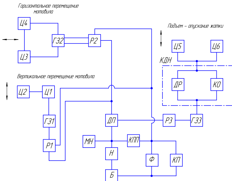
Рис.3 – Структурная схема гидросистемы жатвенной части комбайна «Дон-1500Б»: Б – бак ( W = 25 л), Н – насос шестеренный НШ-32-3, КПП – клапан предохранительно-переливной, P1, P2, P3 – гидрораспределители с механическим приводом (секционные), ГЗ1 – клапан запорный двухстороннего действия (гидрозамок двухсторонний), ГЗ2, ГЗ3 – клапан запорный одностороннего действия (гидрозамок односторонний); КДН – клапан дросселирующий настраиваемый, ДР – дроссель, КО – клапан обратный, Ц1, Ц2, Ц3, Ц4 – гидроцилиндры специальные (двухстороннего действия), Ц5, Ц6 – гидроцилиндры плунжерные одностороннего действия, ДП – делитель потока, КП – клапан предохранительный, Ф – фильтр, МН – манометр.
