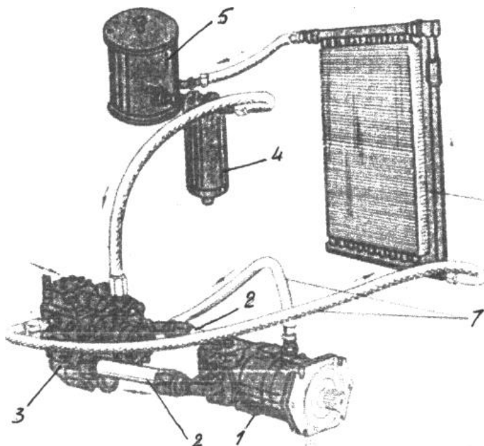
Рис.1. Монтажная схема объемного гидропривода «ГСТ-90»: 1 - аксиально-плунжерный гидромотор; 2 - рукав высокого давления; 3 - аксиально-плунжерный насос; 4 - масляный фильтр; 5 - масляный бак; 6 - масляный радиатор; 7 - дренажные трубопроводы.
