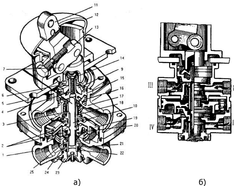
Рис.3 Пневматический тормозной кран: 1- нижний корпус; 2- уплотнительное кольцо; 3,16,21,25- пружины; 4- винт; 5- опорная плита; 6- тарелка пружины; 7- ось рычага; 8- верхний клапан; 9- уравновешивающий элемент; 10- шток; 11- рычаг; 12-уплотнитель; 13- ролик; 14-толкатель; 15- верхний поршень; 17- верхний корпус; 18- верхний клапан; 19- большой поршень; 20- малый поршень; 22- опорное кольцо; 23- выпускное окно; 24- нижний клапан
