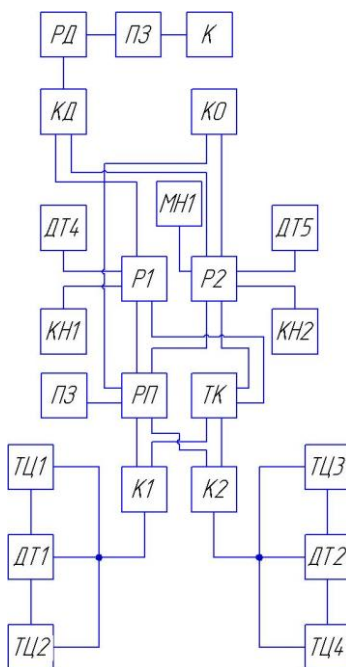
Рис.4 –Схема структурная пневмосистемы автогрейdera ДЗ-98:
