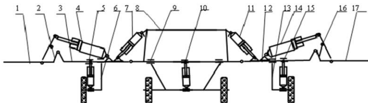
Рис.4 – Упрощенная схема беспсепочного культиватора КШУ-12: 1,17- крайние секции; 2,16-рычажный механизм, 3,12-средние секции,4,14- гидроцилиндры сворачивания крайних секций, 5,10,15- гидроцилиндры выглубления рабочих органов; 6,9,13- механизм подката колес; 7,11-гидроцилиндр сворачивания средних секций; 8 - центральная секция культиватора
