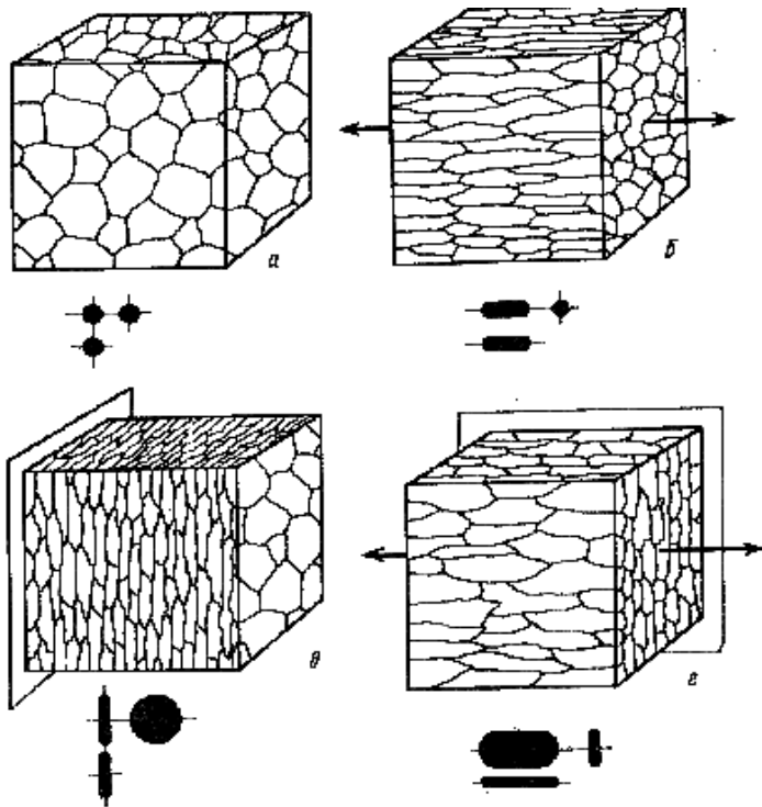
Рис. 5 Классификация граничных поверхностей по видам ориентации и форма микрочастиц: а – изометрическая; б – линейная; в – плоскостная; г –плоскостно-линейная ориентация. Показаны оси и плоскости ориентации
