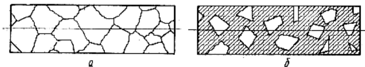
Рис. 26 Образование хорд при пересечении граничных поверхностей однофазной (а) и двухфазной (б)
