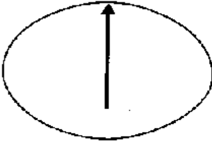
Рис. 19 Секущий линейный контур, составленный из двух арок циклоиды. Периметр контура равен учетверенной длине его малой оси (А.Г. Спектор)
