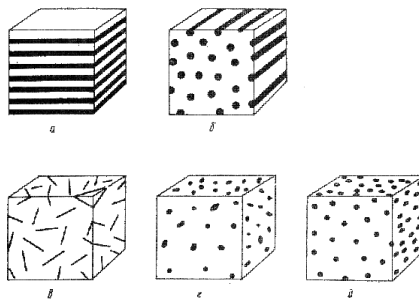
Рис. 3 Классификация эвтектик (эвтектоидов) по геометрии их строения:
