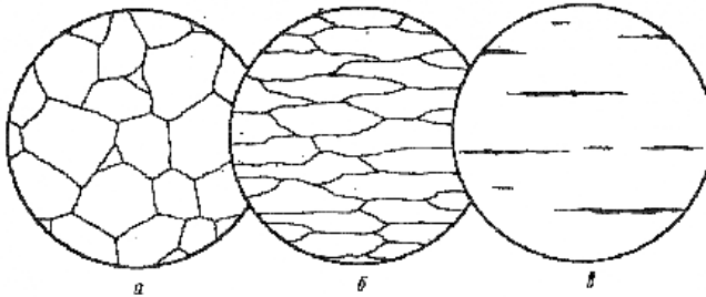
Рис. 4 Различные виды граничных поверхностей: а – изометрические граничные поверхности; б – частично ориентированные; в – почти полностью ориентированные
