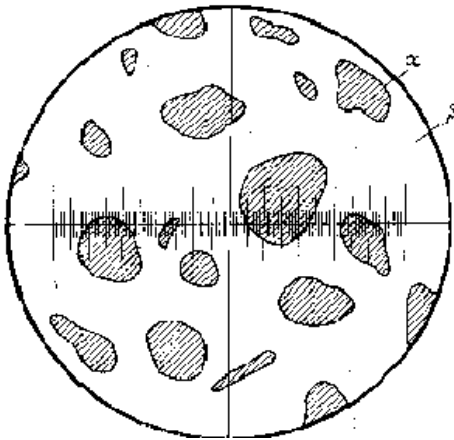
Рис. 16 Схема определения объемной доли фазы \alpha линейным методом при неподвижном шлифе
