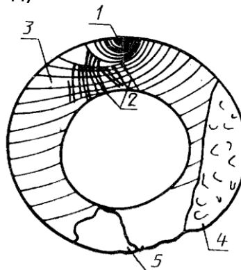
Рис.7. Схема усталостного излома: 1- очаг разрушения, 2- ступеньки и рубцы, 3- усталостные линии, 4- зона ускоренного развития трещины, 5- зона долома
