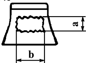
Рис.4. Схема измерения площади хрупкого разрушения в изломе образца
