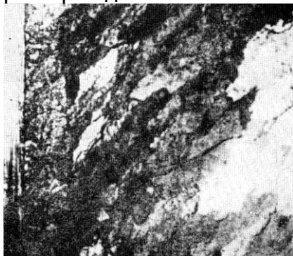
Рис.1. Волокнистый вязкий излом стали
