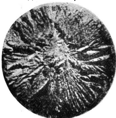
Рис. 2. Хрупкий излом
