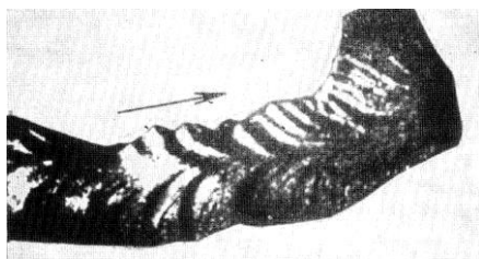
Рис.6. Шевронный усталостный излом, характеризующийся наличием системы ступенек ("елочек" или шеврона)
