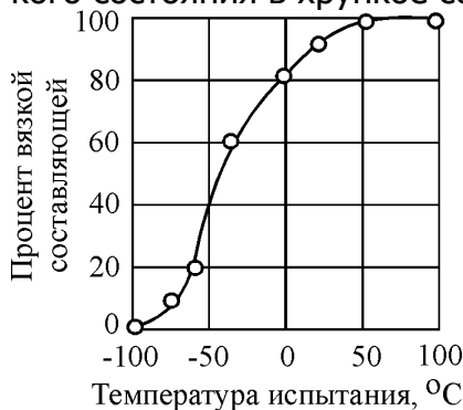
Рис.5. Сериальная кривая вязкой составляющей в изломе стали 40
