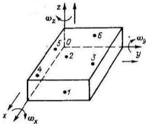
Рис. 7 Базирование детали типа "прямой параллелепипед"
