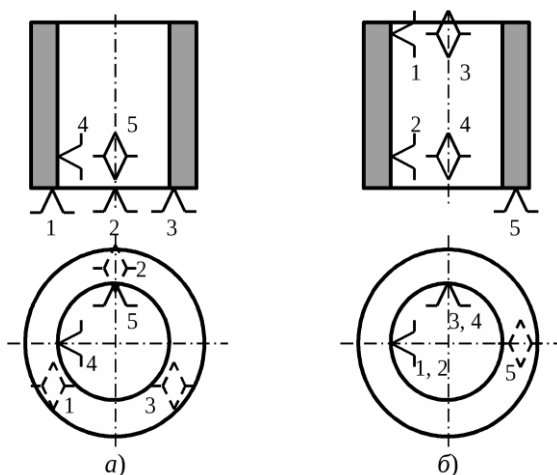
Рис. 10 Варианты (а и б) схемы базирования детали типа "втулка"
