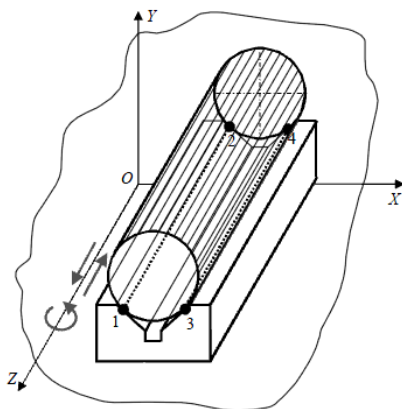
Рис. 4 Двойная направляющая база
