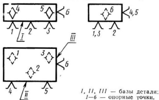
Рис. 9 Схема базирования детали типа "прямой параллелепипед"
