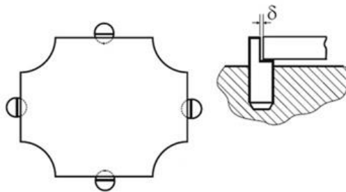
Рис. 12 Упрощенная установка на штифтах детали с большим допуском
