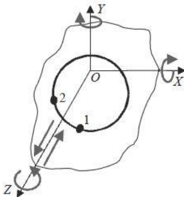
Рис. 6 Двойная опорная база
