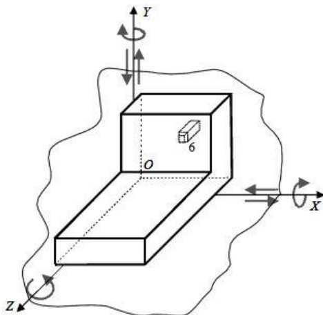
Рис. 5 Опорная база
