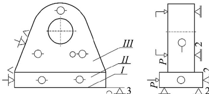
Рис. 12 Принципиальная схема приспособления для сборки проушины
