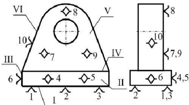
Рис. 11 Схема базирования сварной проушины в сборе.
