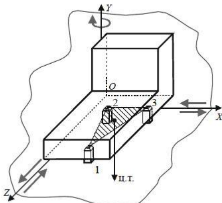
Рис. 2 Установочная база
