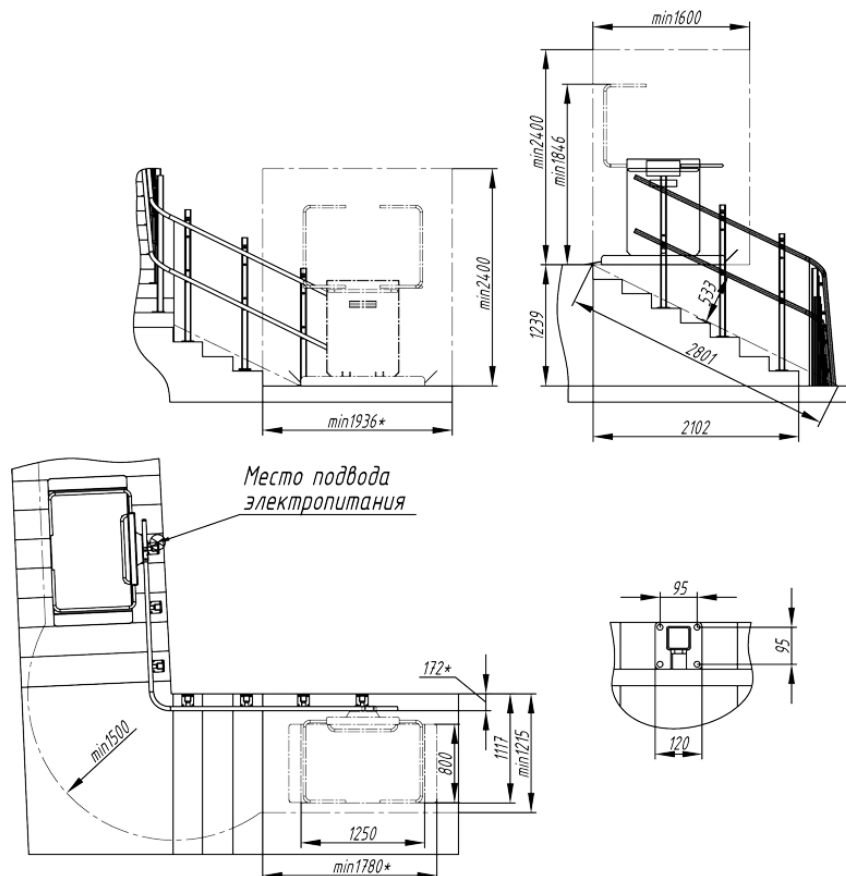
Рис.12. Наклонный подъемник «Инвапром А310»
