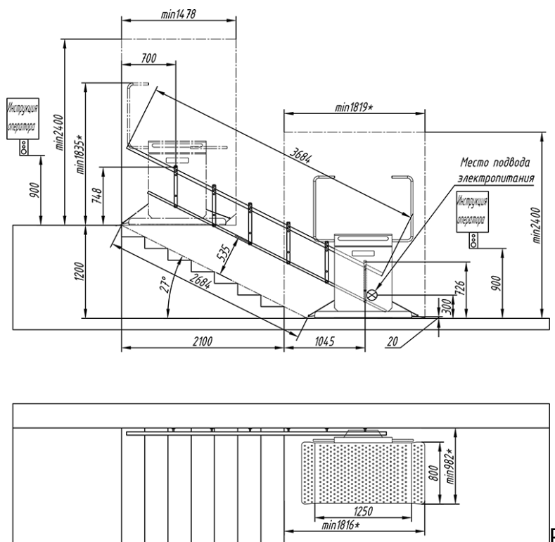
Рис.10. Наклонный подъемник «Инвапром А300»
