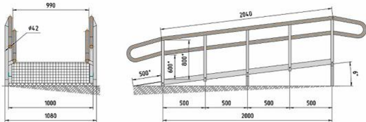
Рис. 13. Стационарный пандус
