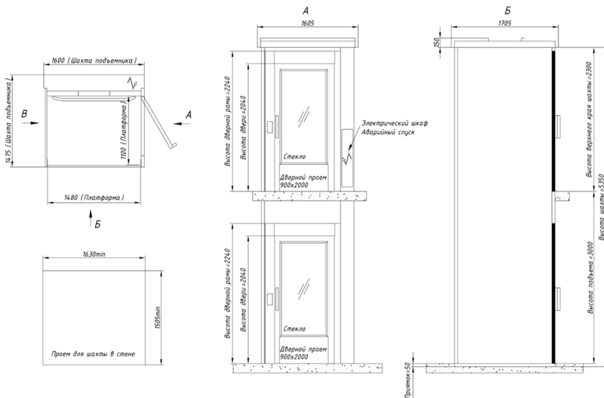
Рис.8. Вертикальный подъемник с шахтой «Инвапром А1»
