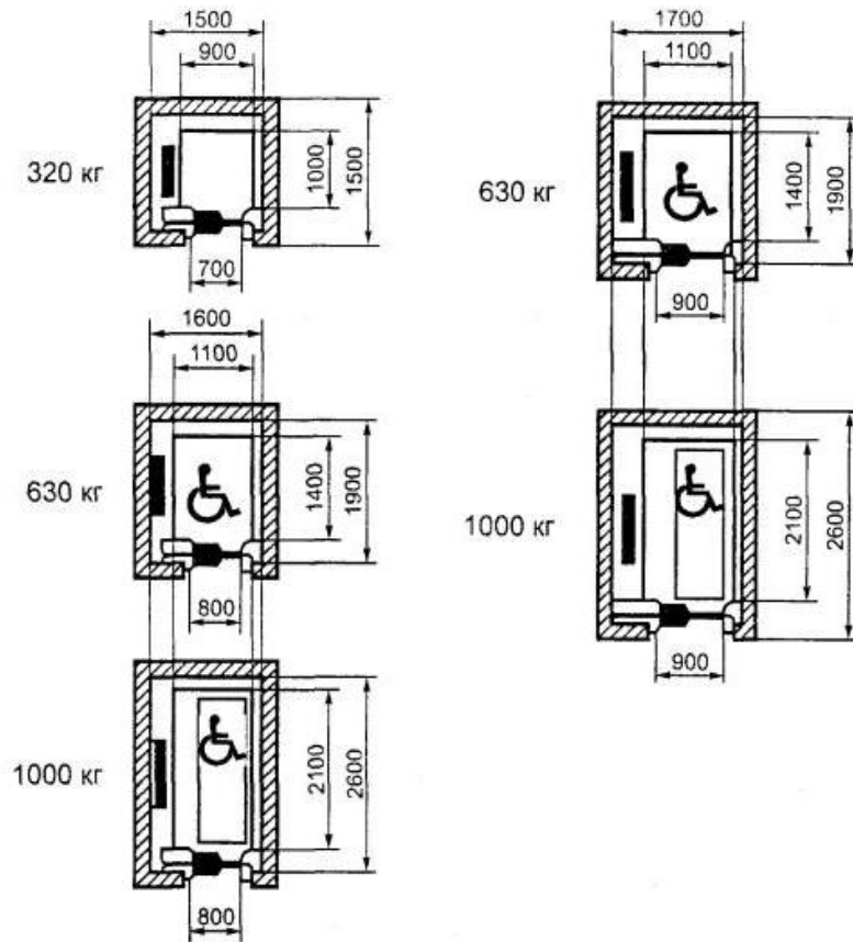
Рис. 3. Пассажирские лифты для жилых зданий
