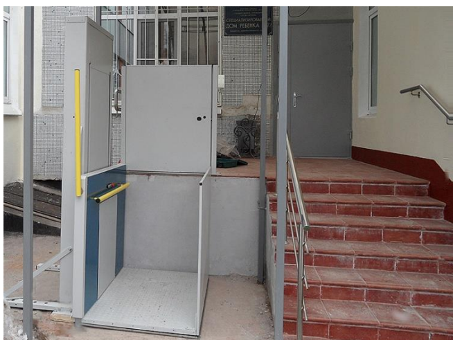
Рис.5. Вертикальный платформенный подъемник «Мультилифт»
