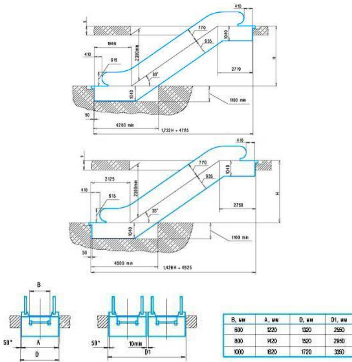
Рис. 14. Конструкция эскалатора
