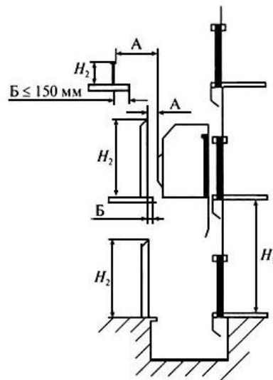
Рис. 1. Расстояние до движущихся элементов лифта
