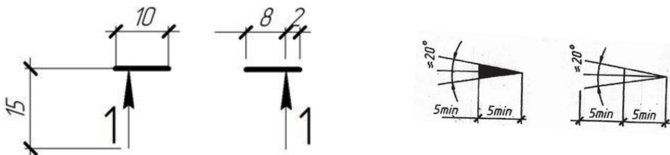
Рис. 16. Начертание стрелок, указывающих направление взгляда
