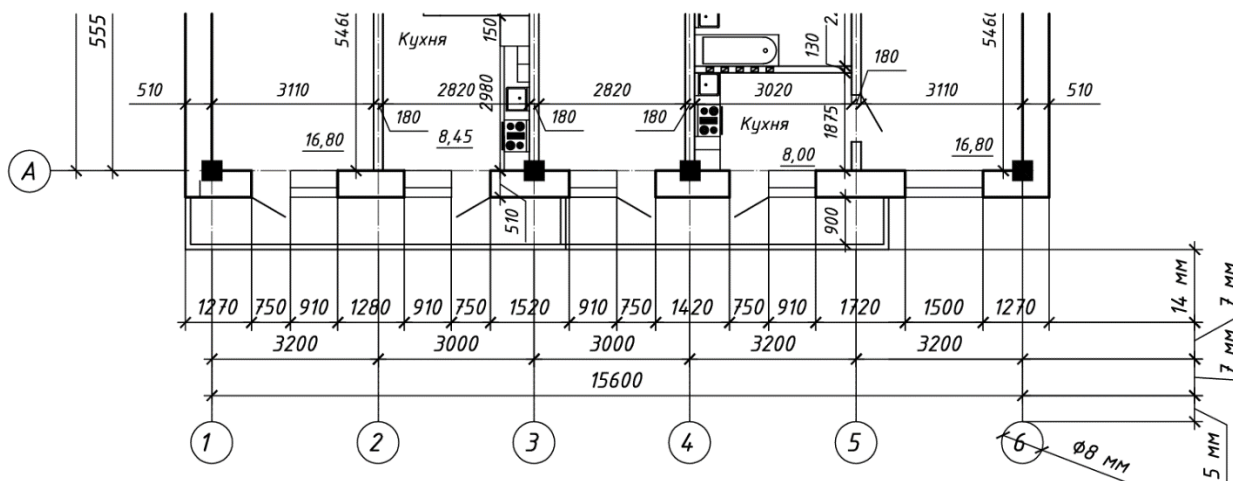
Рис. 7. Рекомендуемое расстояние между размерными линиями
