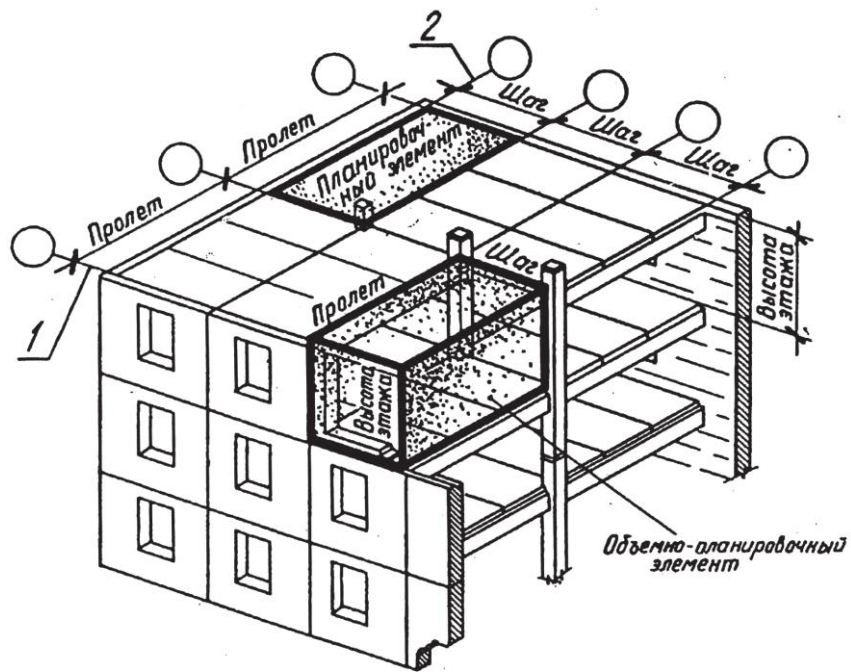
Рис. 4. Объемно-планировочный элемент
