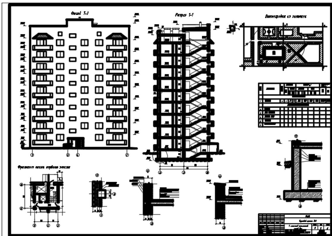
Рис. 25. Пример компоновки чертежей на листе
