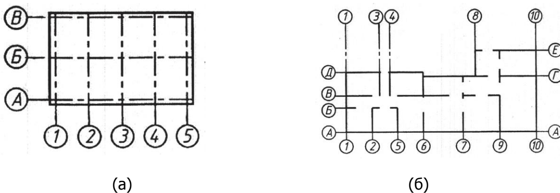
Рис. 5. Обозначение координационных осей
