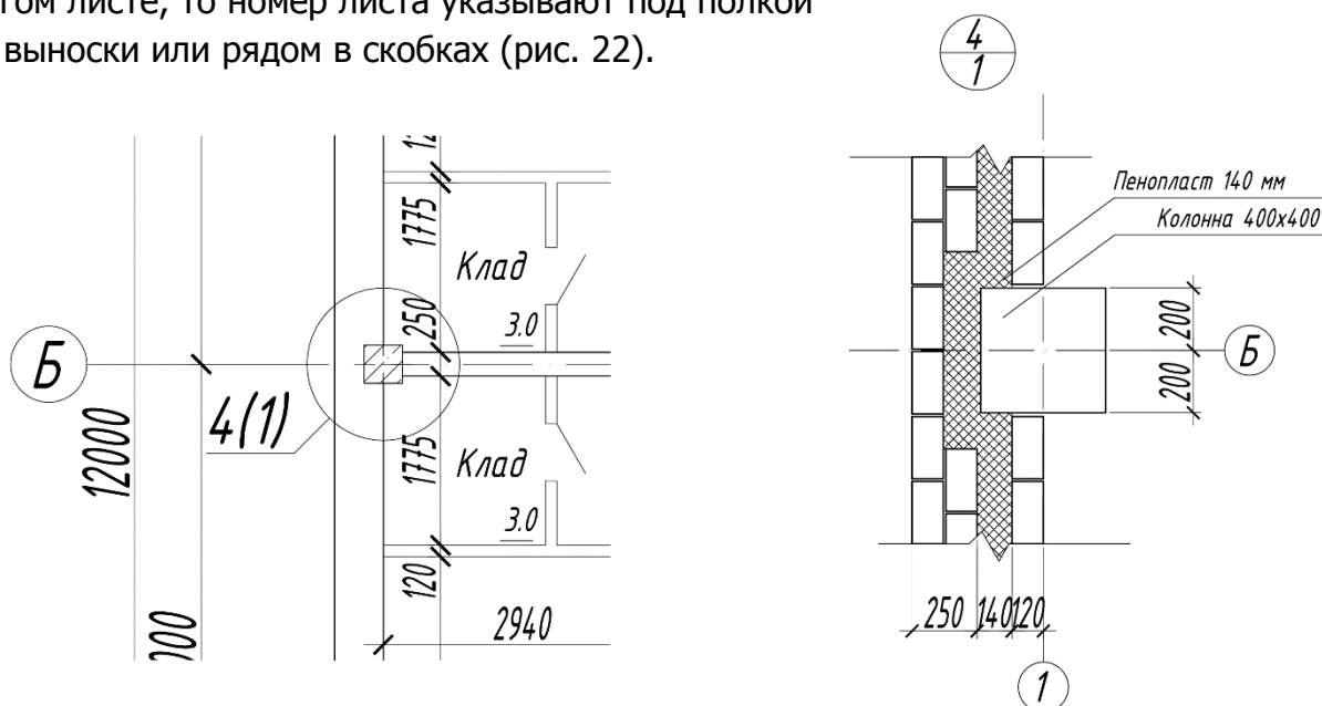
Рис. 22. Пример изображения узла
