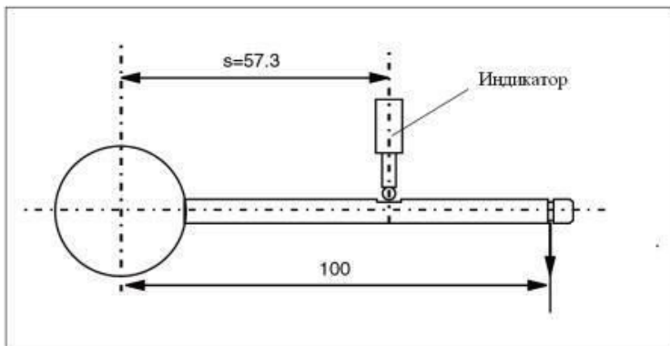
Рис. 2. Рычаг для создания крутящего момента
