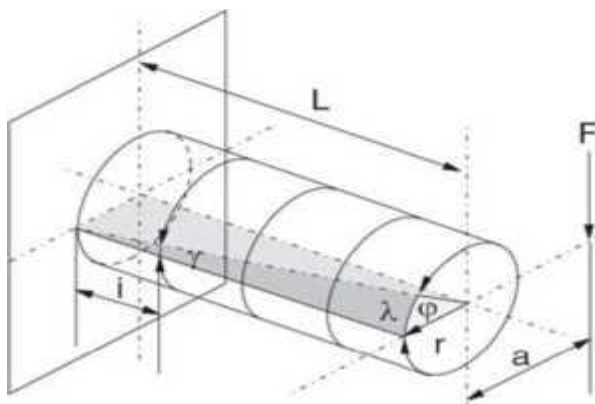
Рис. 5. Испытание стержня на кручение На этом рисунке:
