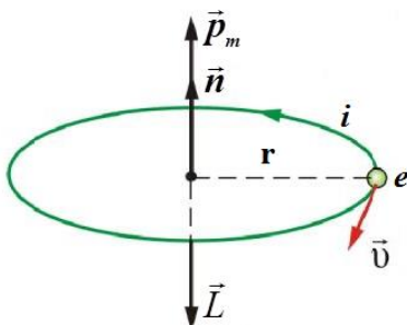
Рисунок 3- Орбитальный магнитный и механический моменты электрона
