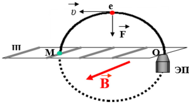
Рисунок 2 – Траектория движение электрона в однородном магнитном поле по окружности
