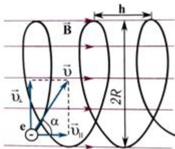
Рисунок 1 - Траектория движение электрона в однородном магнитном поле по винтовой линии
