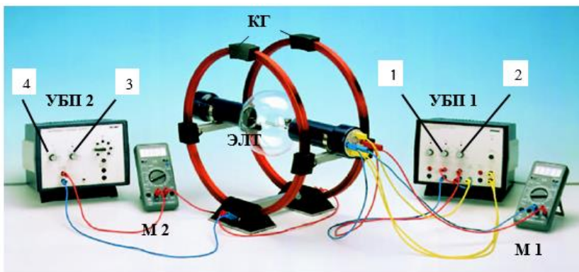
Рисунок 4 - Экспериментальная установка
