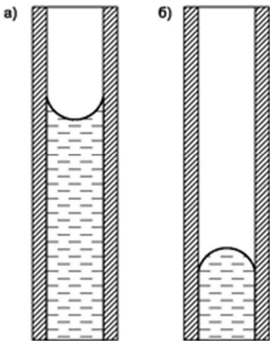
Формы менисков
