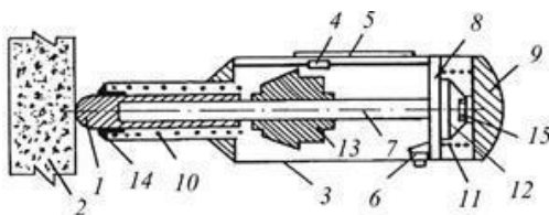
Рис. 3. Прибор Шмидта типа N
