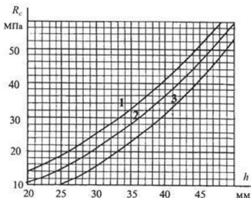
Рис. 4. Графики зависимости величины отскока бойка прибора Шмидта от прочности бетона при различном положении прибора: 1 – вертикально вниз; 2 – горизонтально; 3 – вертикально вверх
