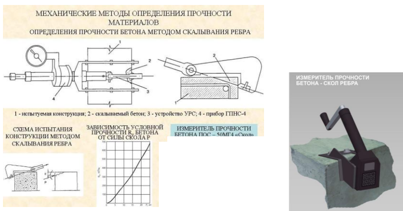
Рис. 6. Определение прочности бетона методом скалывания ребра
