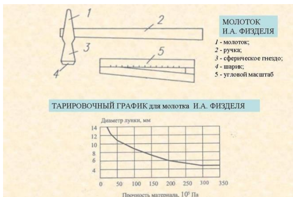
Рис. 1. Молоток И.А. Физделя
