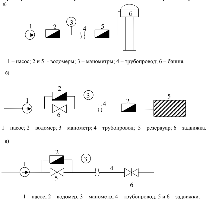
Рис. 54. Схемы определения величины утечки
