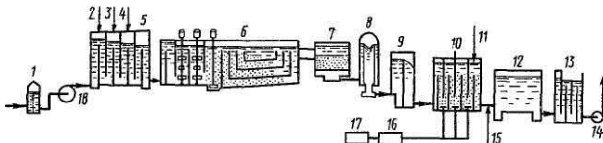
Рис. 3.23. Технологическая схема подготовки воды на станции Нейлисюр-Марн (Франция):
