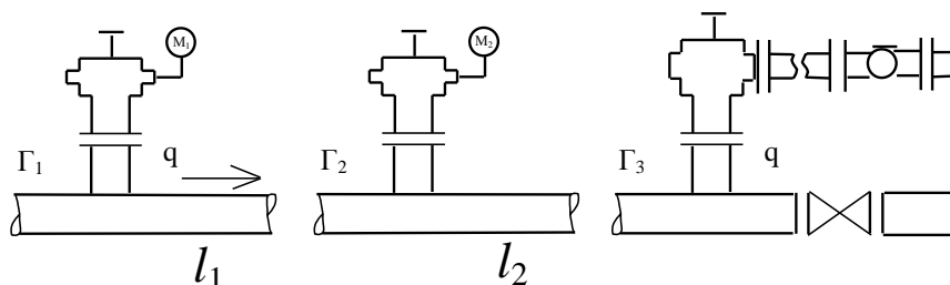
Рис. 52.Схема гидравлического испытания трубопровода
