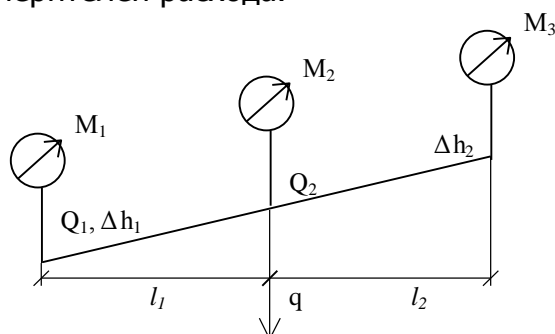
Рис. 53. Принципиальная схема испытания методом трех манометров
