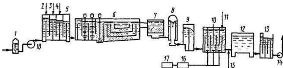
Рис.6. Технологическая схема подготовки воды на станции Нейлсюр-Марн (Франция):
