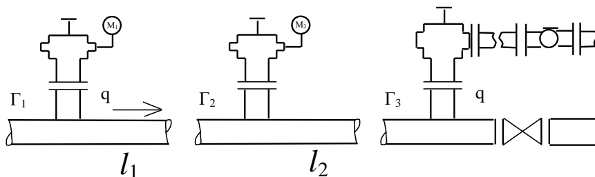
Рис. 2.Схема гидравлического испытания трубопровода
