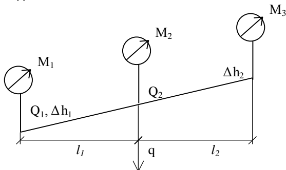
Рис. 3. Принципиальная схема испытания методом трех манометров
