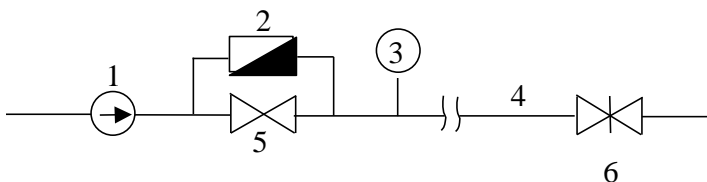
Рис. 5. Схемы определения величины утечки
